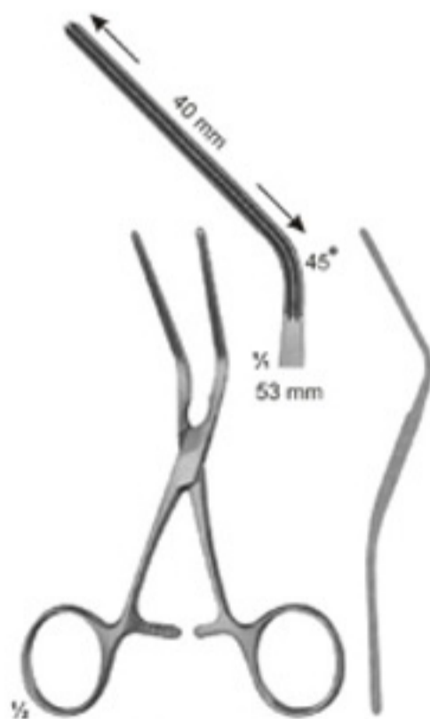
17-173 DE-BAKEY 45° winklig gebogen angled 45° 125 mm
