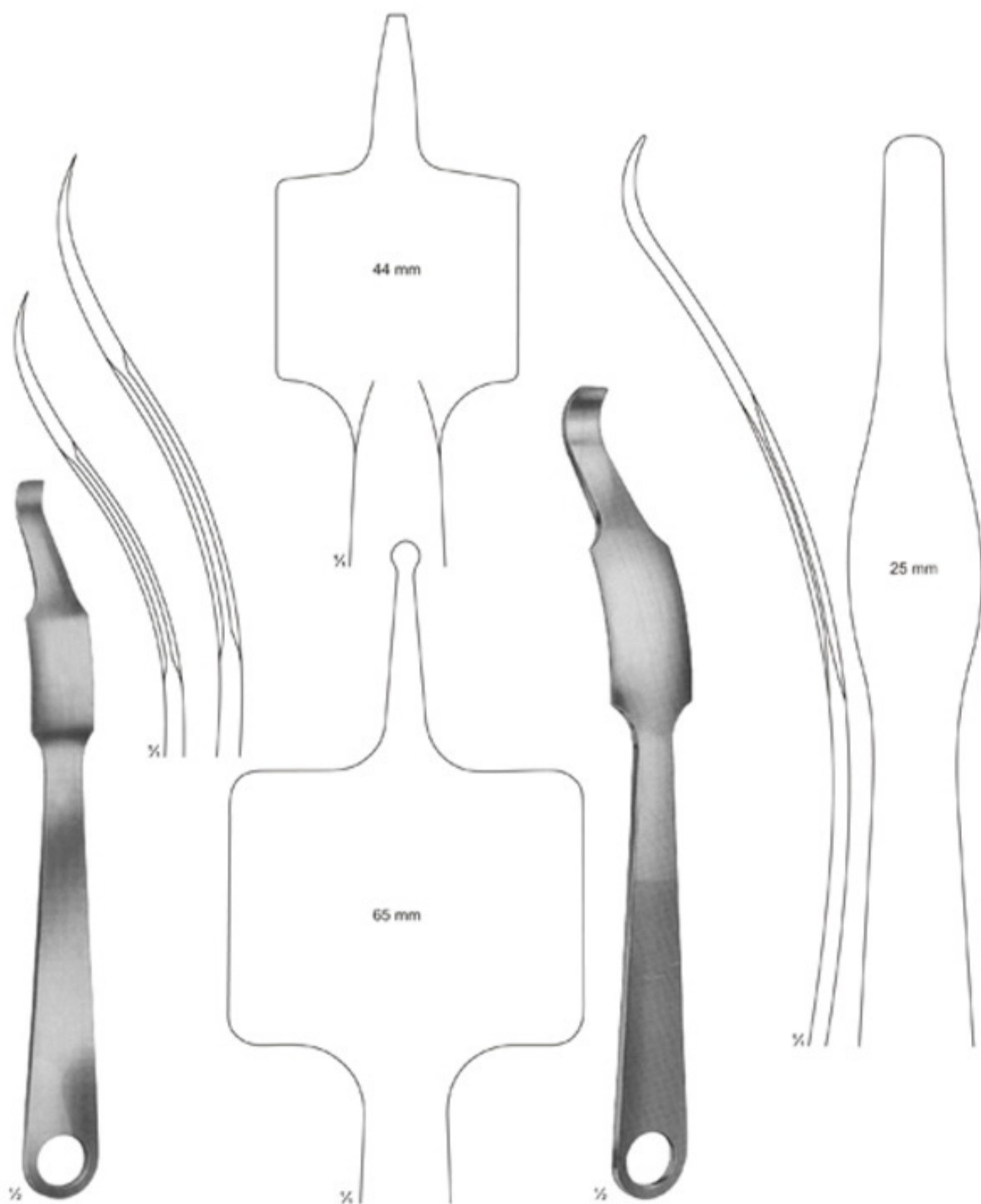
20-125 - 126 VERBRUGGE-MULLER 20-125 240 mm 20-126 255 mm
