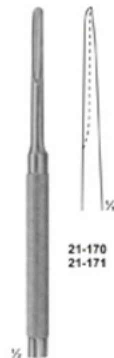
LUCAS 21-170 - 171 Gouges 160 mm
